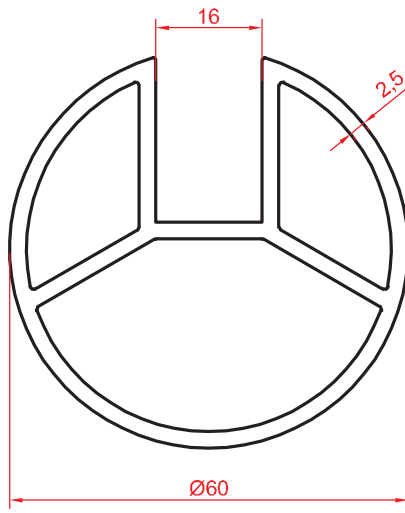
636 1.812 kg/m
