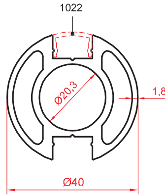
1010 1.143 kg/m
