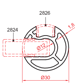
2825 0.598 kg/m
