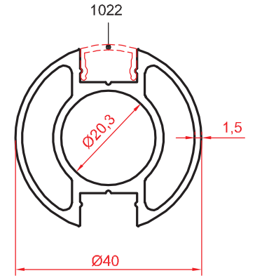
1565 0.911 kg/m
