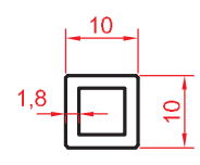
1576 0.160 kg/m
