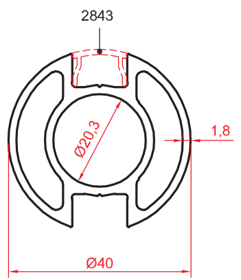
2841 1.002 kg/m
