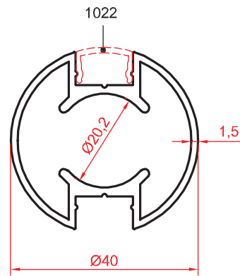
1599 0.762 kg/m
