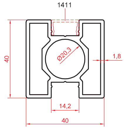
1410 1.188 kg/m
