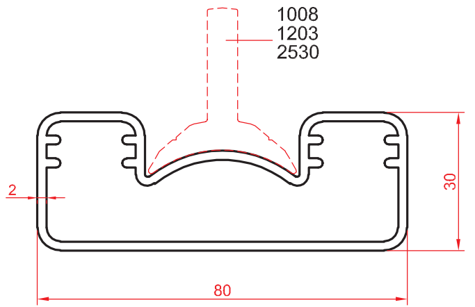
1399 1.374 kg/m
