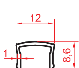
1233 0.074 kg/m
